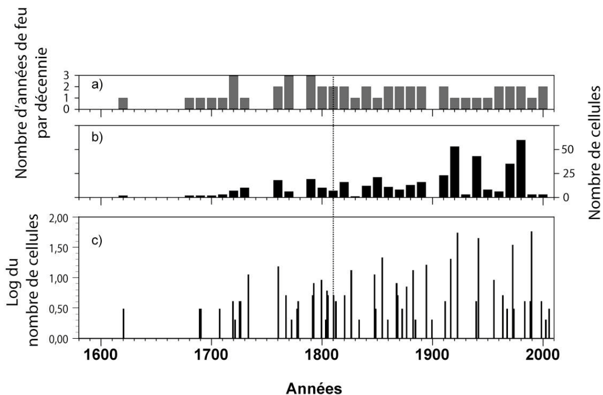
Figure 3. Nombre d'années de feu (a) et nombre de cellules brûlées par décennie (b) et log du nombre de cellules brûlées par année au long du transect étudié. Le trait vertical pointillé indique l'année de 1810 à partir de laquelle on estime que la plupart des feux ont été détectés dans chaque cellule.
