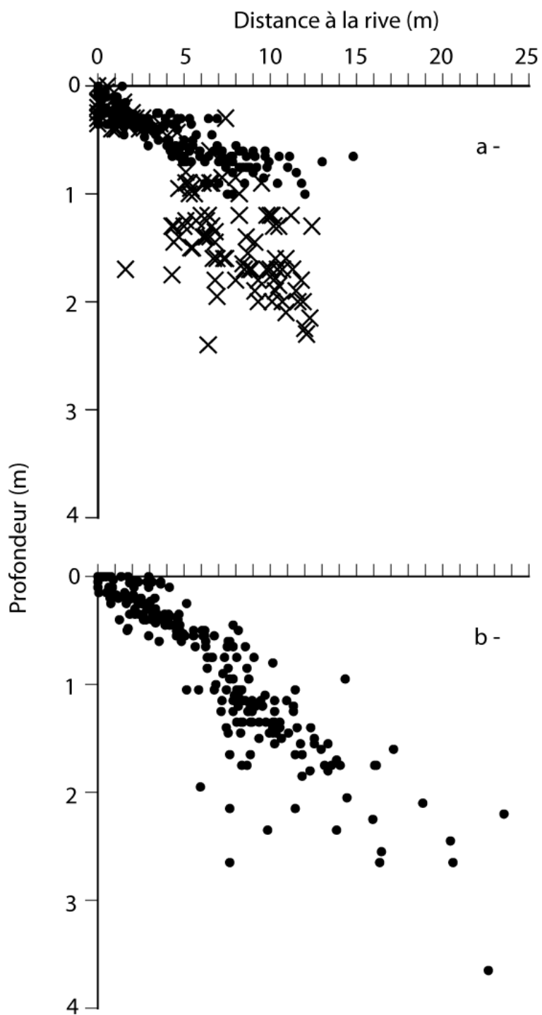
Figure 4. Profondeur des DLG en fonction de la distance à la rive dans la zone littorale du lac I (a) et du lac II (b). Les points et les croix représentent respectivement les spécimens du tronçon 1 et du tronçon 2 au lac I.
